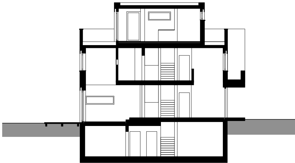
SCHNITT 1 - 1
