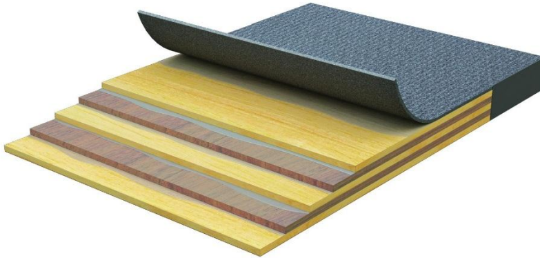
Abbildung 1 VANyCARE® - Schichtaufbau
