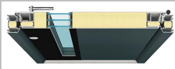
Abb_01: foradur made by puren ist eine Entwicklung für die speziellen Anforderungen der Haustürproduktion. Abbildung: puren
