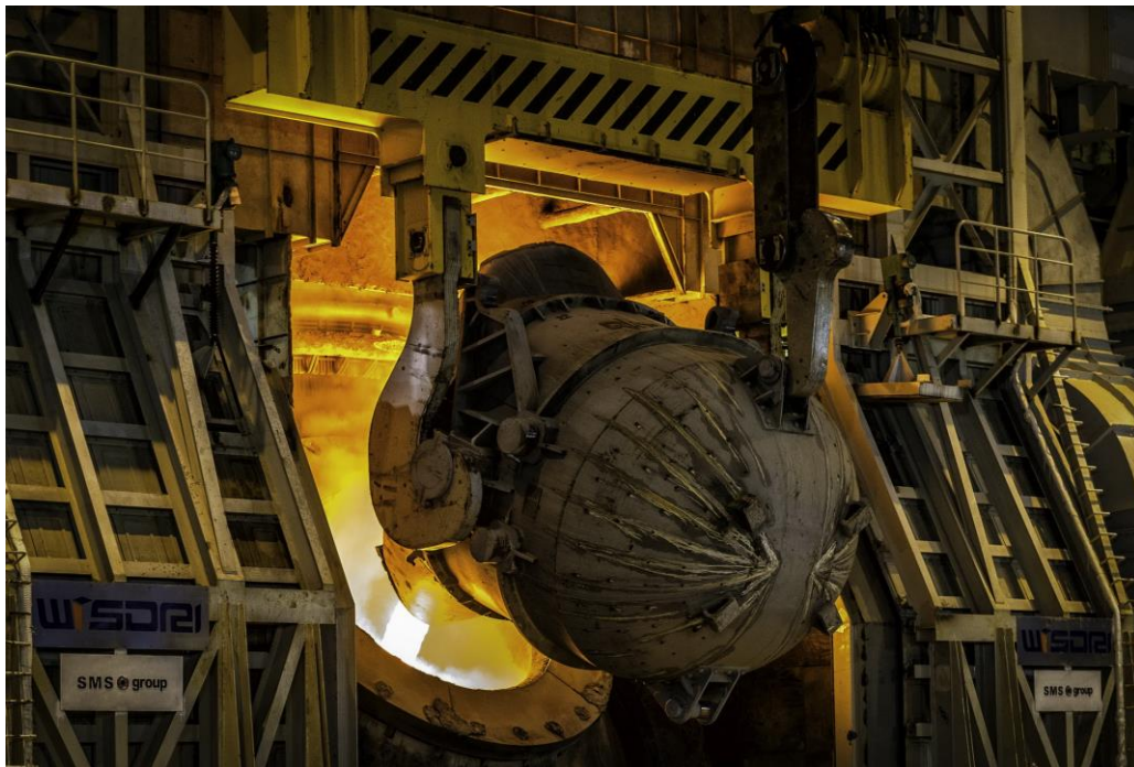
Erste Schmelze von Konverter Nr. 2 bei Hoa Phat, Vietnam.
