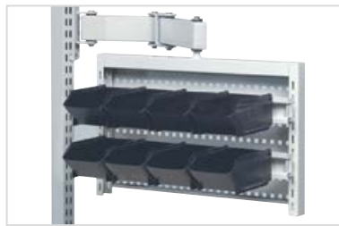
Drehbarer Universalhalter mit Lochblech M500, Aufhängeleiste M500 und 8 Kunststoffkästen ESD
