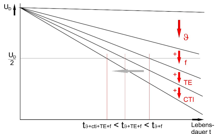
Reduktion der möglichen Einsatzdauer durch Reduktion der Durchschlagsspannung aufgrund von Temperatur, Frequenz, Teilentladung (elektrischer Stress) und Umweltbedingungen (Quelle: CMC)
