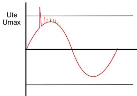
Getriggert TE-Einsatz durch Überspannungsimpuls auch unter TE-Einsatzspg.
