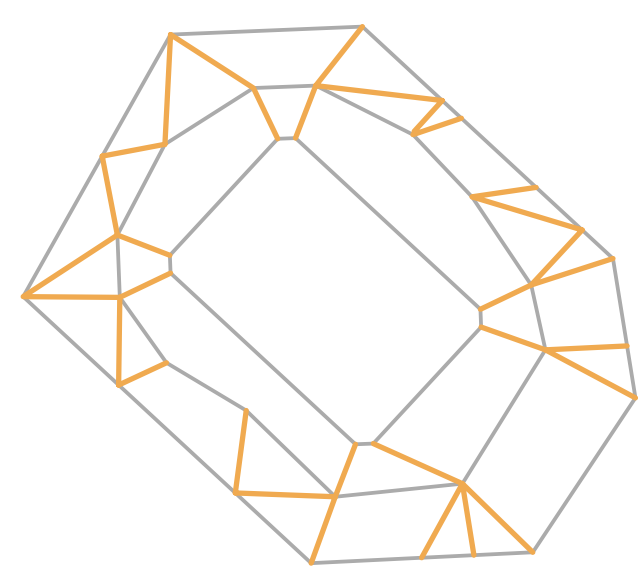
Fachwerkträger
