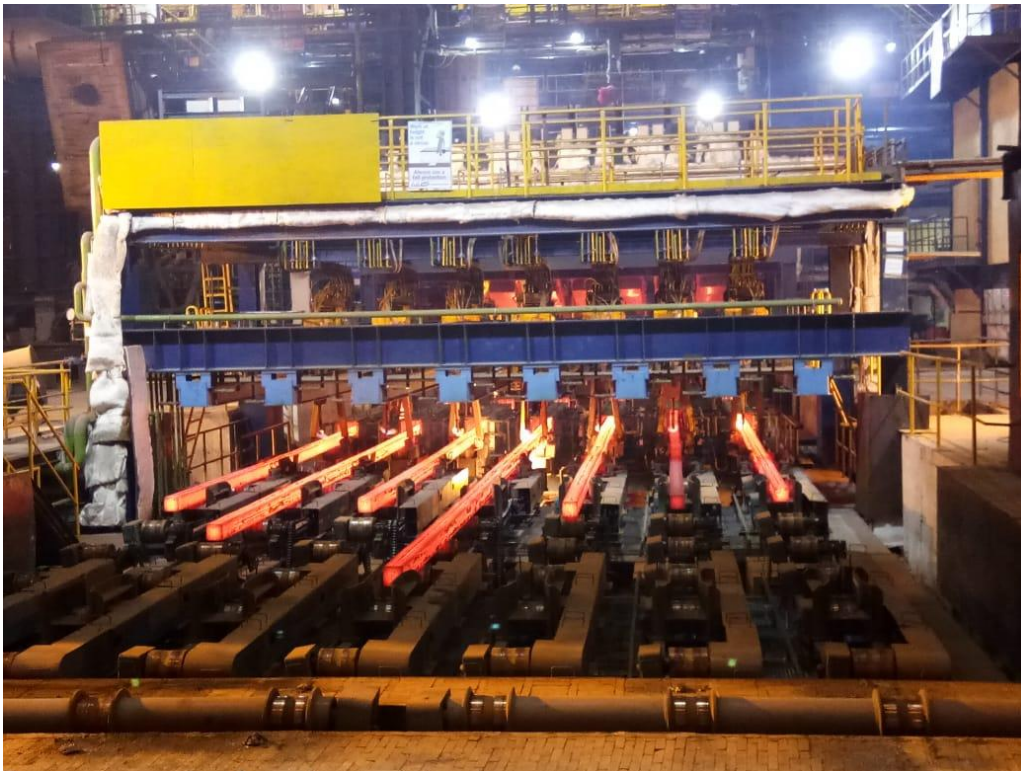
Neue Hochgeschwindigkeits-Kombi-Stranggießanlage mit sieben Strängen in Betrieb bei JSPL Angul.
