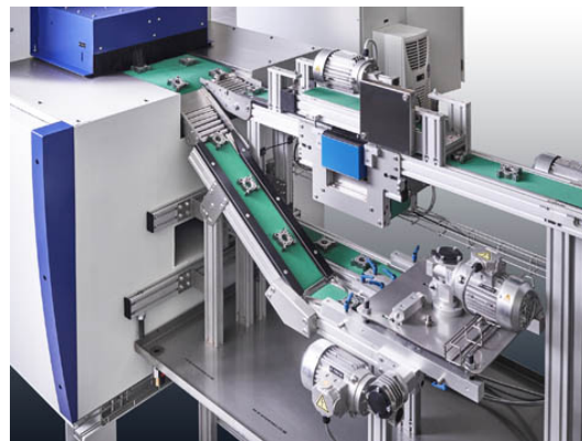
Bild Nr. 08-10 SY-Wendeeinheit.jpg.
