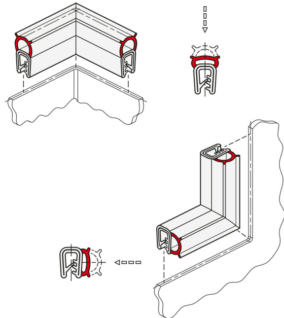
GN 2181 Kantenschutz-Dichtprofil-Ecken – oben Form A, unten Form D
