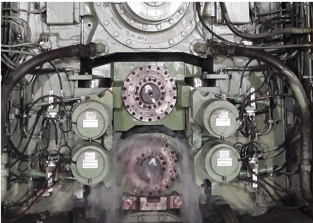
Fertigerüst F4 der Warmbandstraße bei WISCO nach dem Einbau des CVC®plus-Systems.
