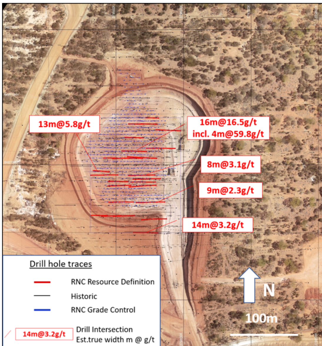
Abbildung 4: Fairplay North Stage 1 Planansicht mit Bohrungen 2019 RNC
