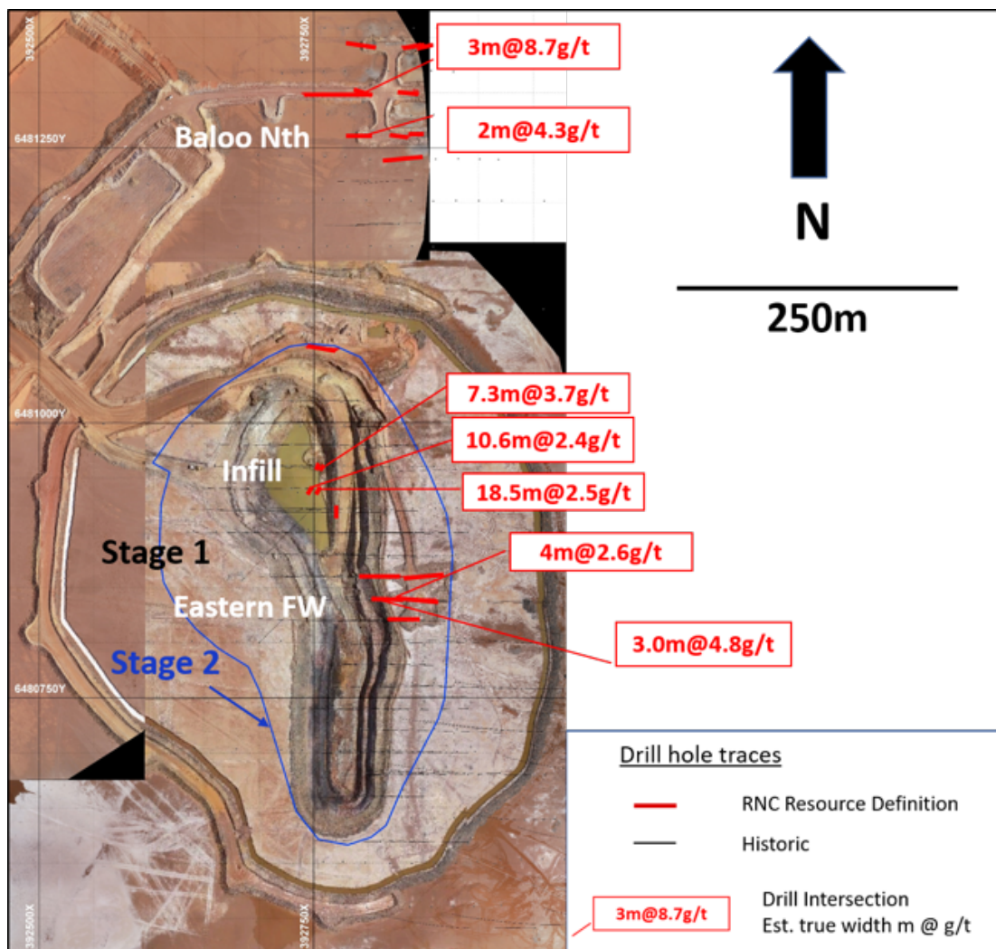
Abbildung 2: Planansicht von Baloo mit den Bohrungen im Jahr 2019 und dem geplanten Entwicklungsplan der Phase 2.
