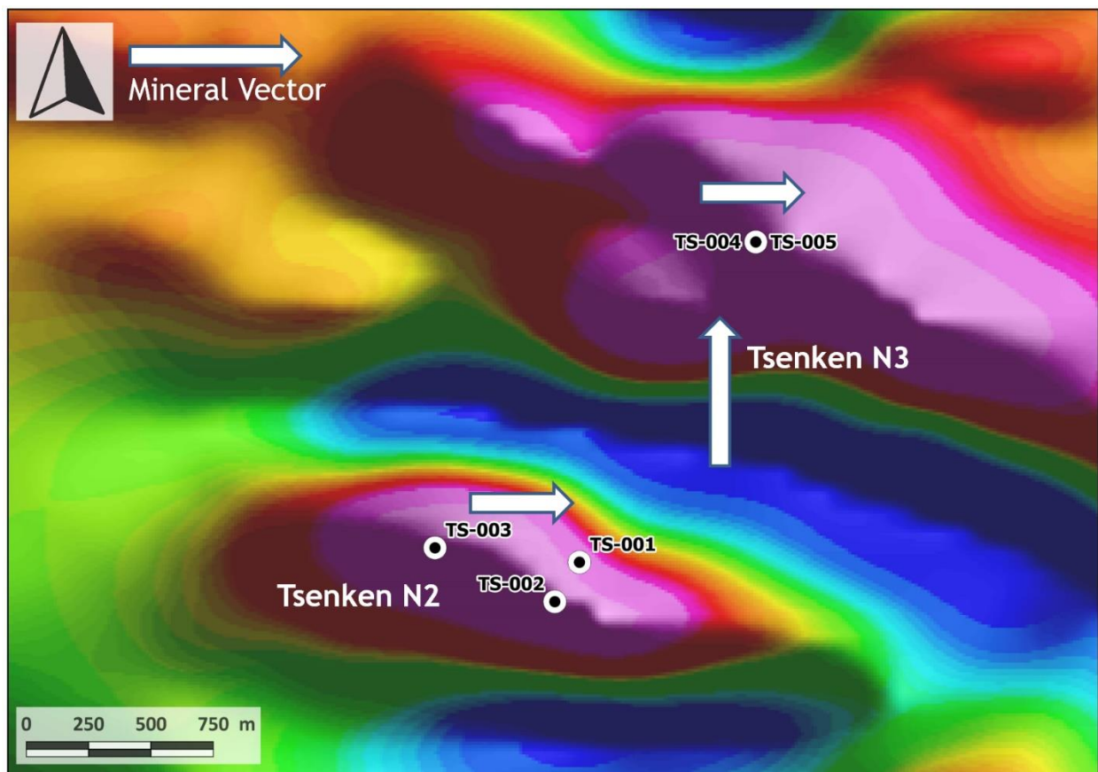
Abbildung 1. Draufsicht der magnetischen Merkmale, die die Hauptziele im Bereich Tsenken N2 und N3 bildeten, mit Darstellung der Bohransatzstellen für TS-001 bis TS-005. Die Pfeile zeigen die Richtung der zunehmenden Alteration und der Kupfervererzung. Die Abbildung des Magnetismus ist die negative Reduktion zum Äquator.
