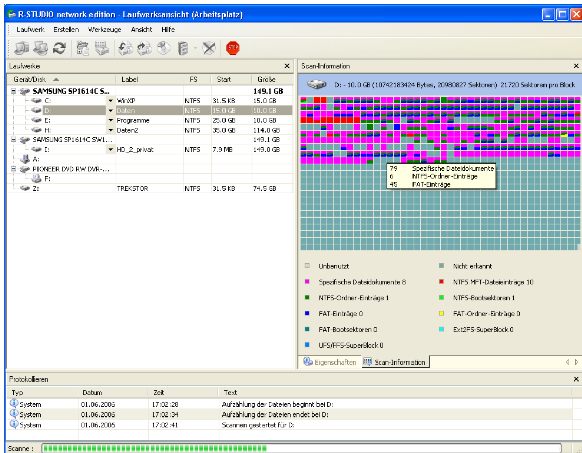
R-Studio 3 beim Scannen einer Partition
