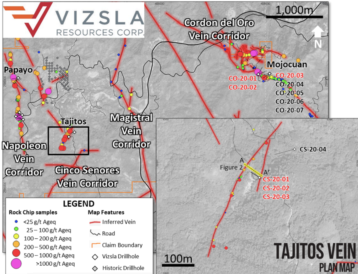
Karte mit Lage der Bohrungen, kartierten Erzgängen sowie Übertageprobenentnahmen im Prospektionsgebiet ‚Tajitos‘ auf dem Gangkorridor ‚Cinco Senores‘ und im Prospektionsgebiet ‚Mojocuan‘ auf dem Gangkorridor ‚Cordon del Oro‘.
