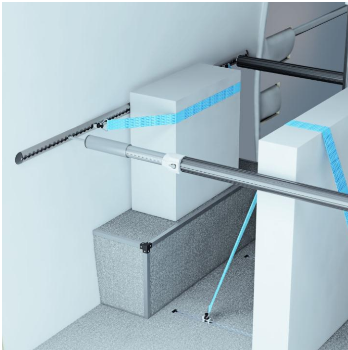
Abbildung 3 VANYCARE®-Komplettausstattung incl. Radkastenverkleidung und Zurrschienen
