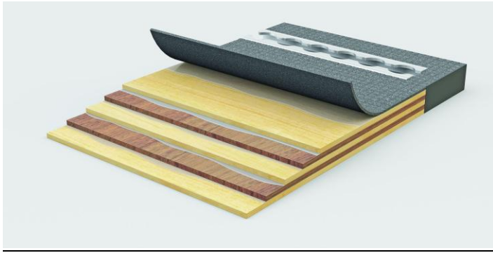
Abbildung 2 Schichtaufbau eines VANYCARE®-Transporterbodens Professional
