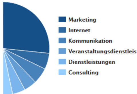
Branchen-Verteilung:
