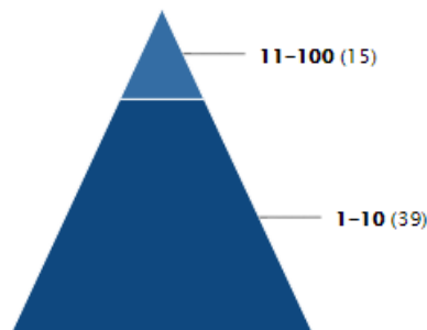
Nach Mitarbeiterzahl
