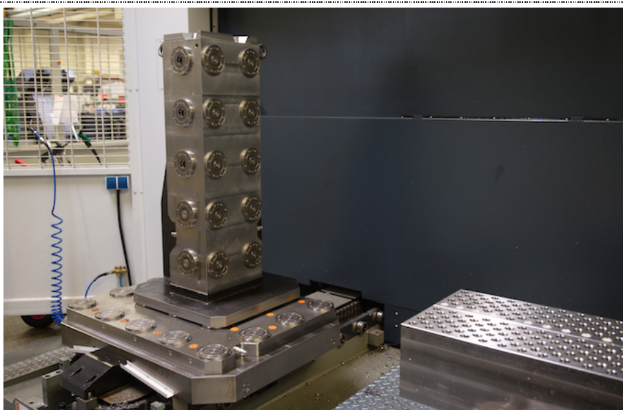
Bild Nr. 125-03 AM_MG-Spannturm.jpg.
