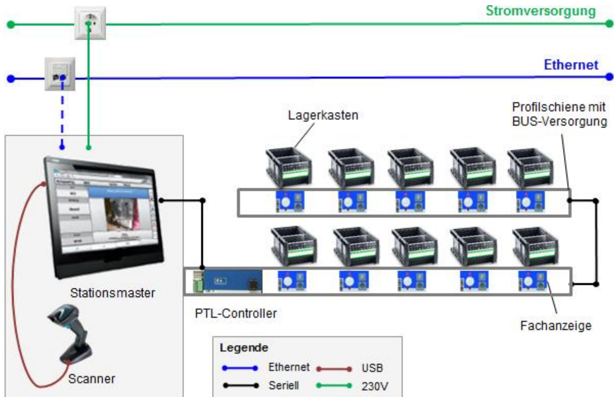
Geräteplan für die Anwendung mit Monitor, Scanner und Pick to Light.
