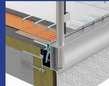
Pfostengeländer AQUA VIVA ORBIS
