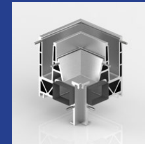
Eckausbildung Außen
