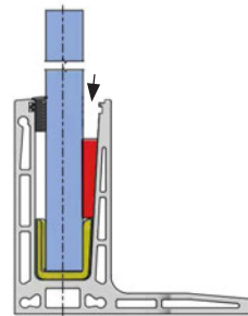
3. Befestigungskeil einsetzen
