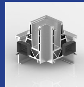
Eckausbildung Innen
