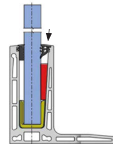
4. Dichtgummi anbringen. Fertig.
