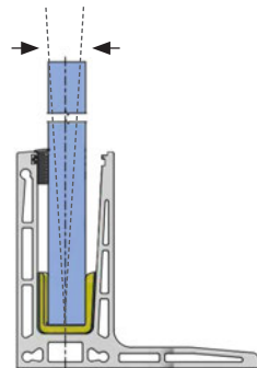
2. Scheibe mit Adjust ausrichten
