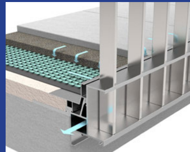
Pfostengeländer AQUA VIVA SIMPLUM
