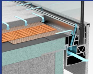
Ganzglasgeländer AQUA VIVA VISIOPLAN
