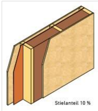
SWISS KRONO Außenwand F60 Brandschutz (Aufbau von innen nach außen)
