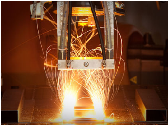
Bild 3: „Remote-Laserstrahlschweißen mit Scanner-Optik“ Bayerisches Laserzentrum GmbH, Markus Weigl, Erlangen*
