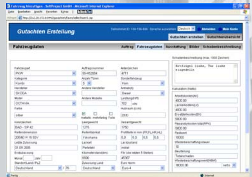
Eingabe Fahrzeugdaten
